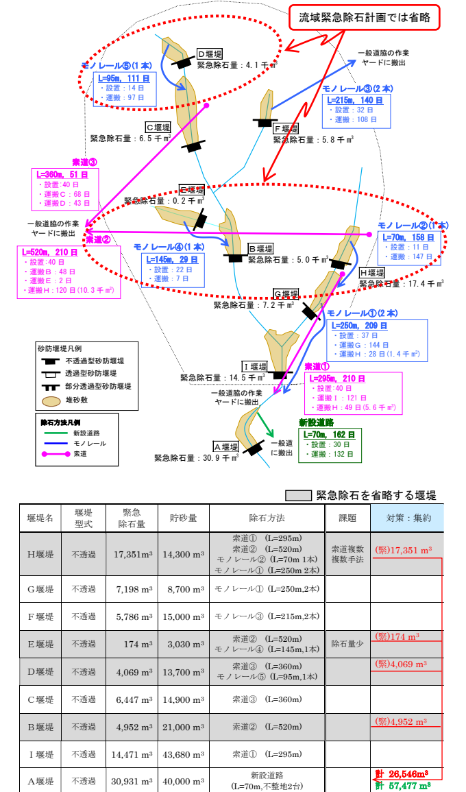
図-3 ゾーンVにおける流域緊急除石方法選定結果
