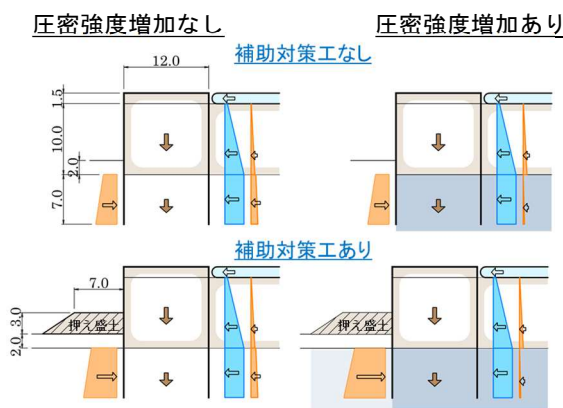
図-5 圧密強度増加有無に対する荷重分布 (非越流部堤体)
