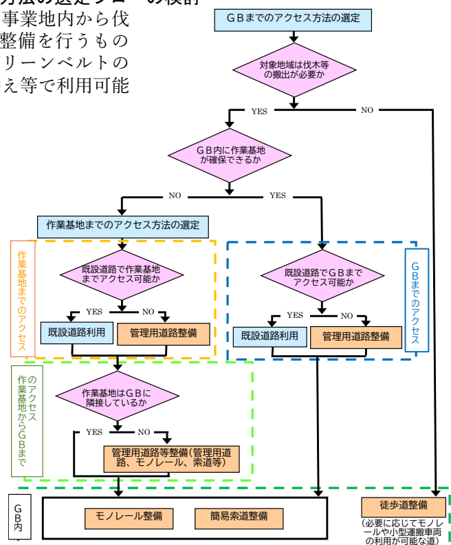
図-2 グリーンベルト（GB）事業地の維持管理のためのアクセス方法の選定フロー（案）
