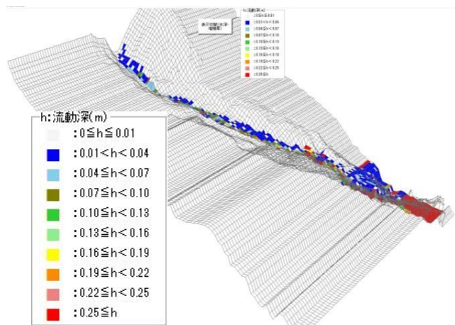
(図 4. 2) 二次元解析結果の例
