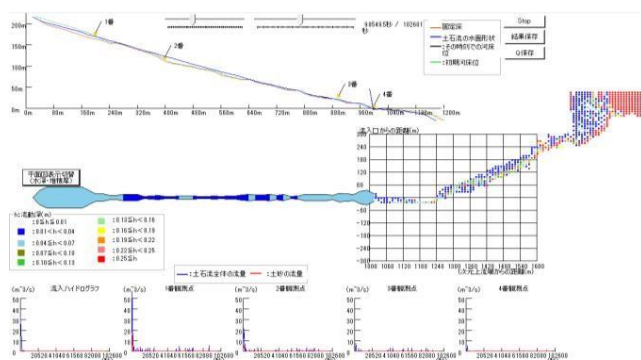
(図 4. 1) 一次元解析結果の例
