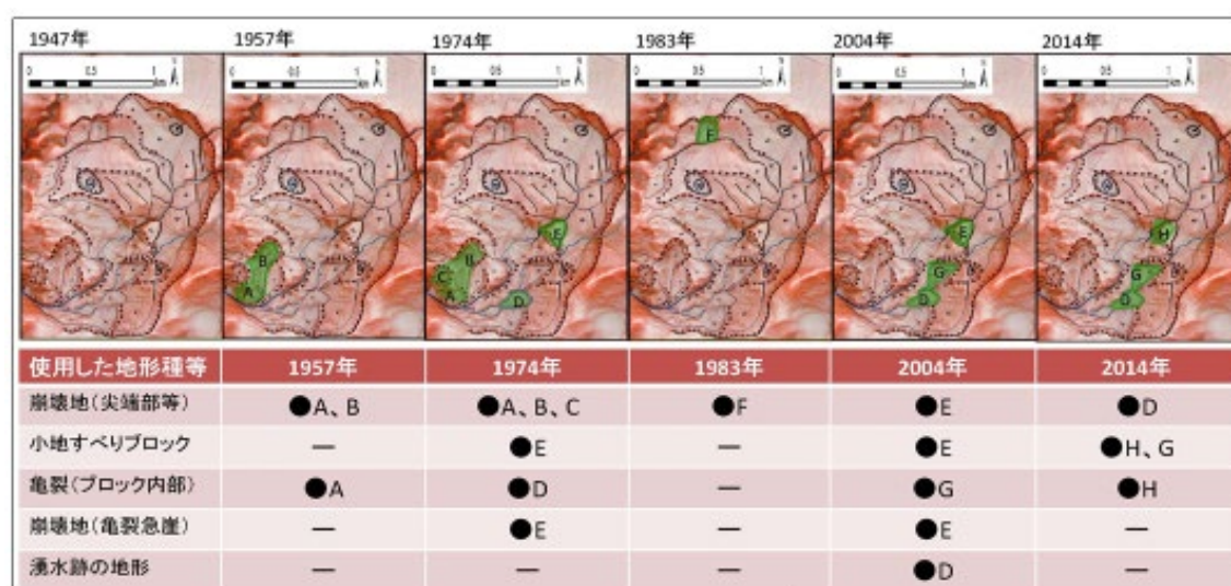
図 2 地すべりブロック活動推移状況図
