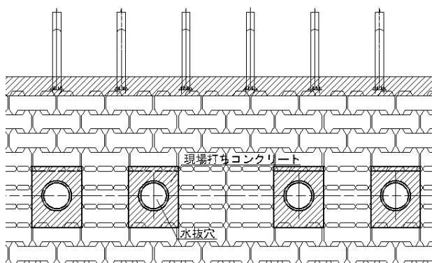
図6 水抜穴の設置
