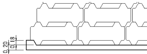
図5 基礎コンクリートの下流端形状
