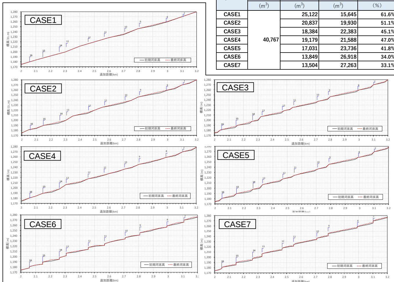
図-7 計算結果
