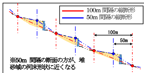
図-5 CASE2, 3の計算断面設定方法
