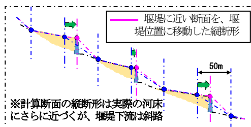
図-6 CASE4, 5の計算断面設定方法
