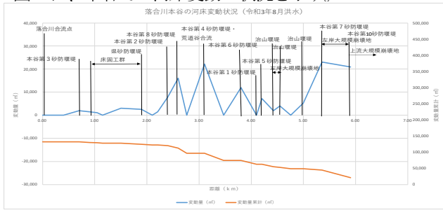
図-4 落合川本谷の河床変動状況
