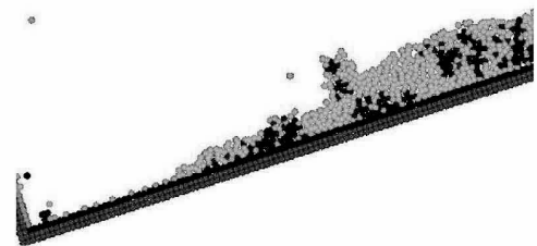
図-8 礫3:砂7の場合のフロント部の状況
