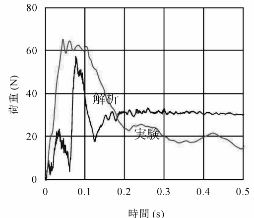
図-7 荷重～時間関係の比較
