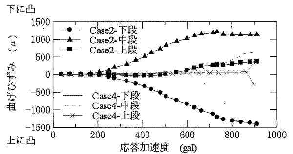
図6 補強材⑩の曲げひずみ(Case2、4)
