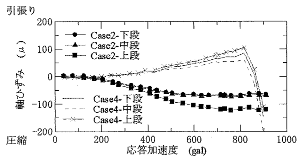
図7 補強材⑩の軸ひずみ(Case2、4)
