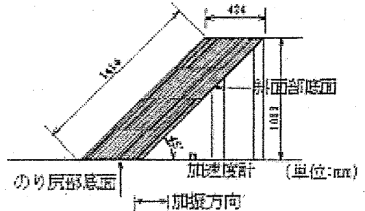
図2 土槽側面図
