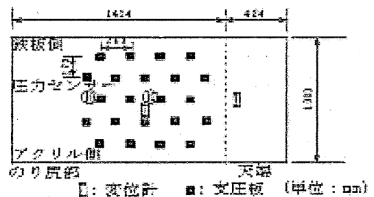
図3 補強材と計測器の配置図
