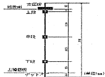
図4 補強材⑩のひずみ計測位置
