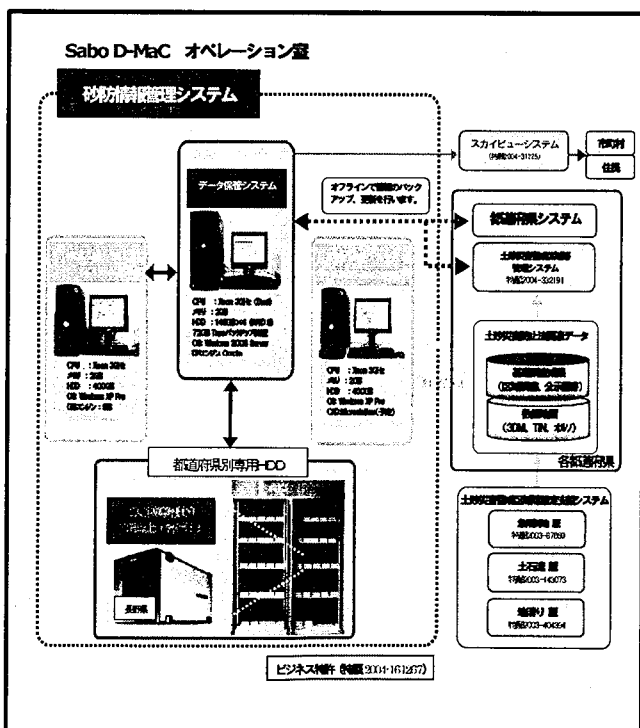
図1 「Sabo D-MaC」の全体像
