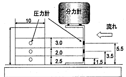
図-2 測定システム
