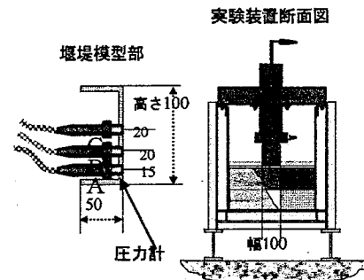
図-1 実験水路 (勾配 1/5)
