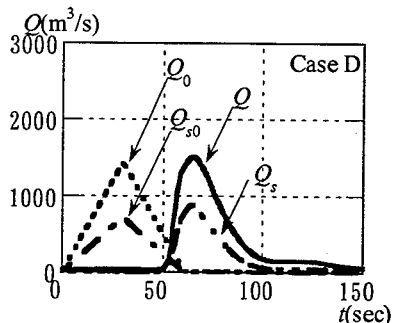
(d) Case D におけるハイドログラフ
