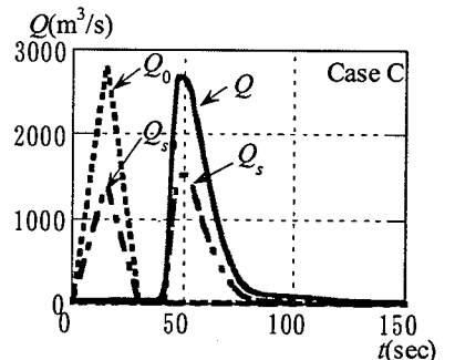
(c) Case C におけるハイドログラフ
