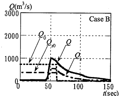
(b) Case B におけるハイドログラフ
