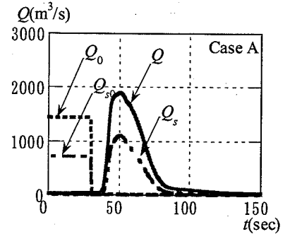
(a) Case A におけるハイドログラフ
