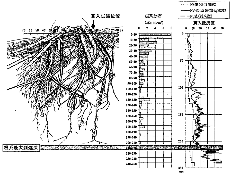
図2 各試験機の貫入抵抗値と根系発達状況の関係 (調査木: H14m コナラ, 土質: 関東ローム層)
