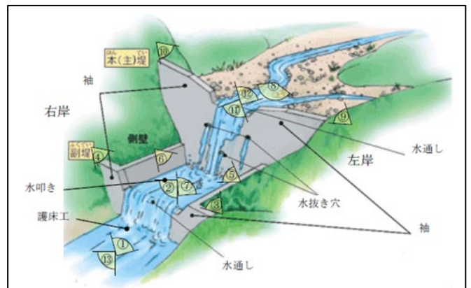
図1 現行点検要領における写真撮影箇所 国土交通省砂防部 (2020) の砂防関係施設点 検要領(案)より引用
