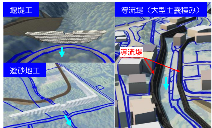
図-1 緊急ハード対策工 統合モデル
