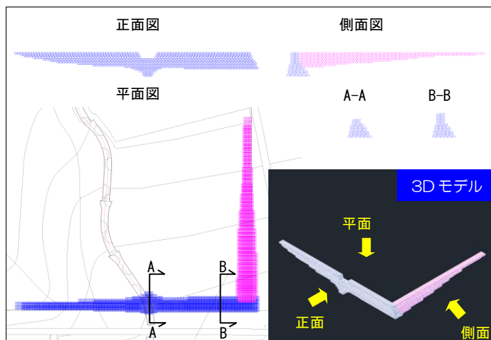
図-5 3次元モデルからの2次元図面作成
