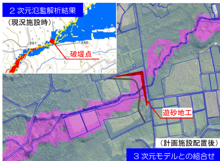
図-4 2次元氾濫解析と3次元モデルの組合せ
