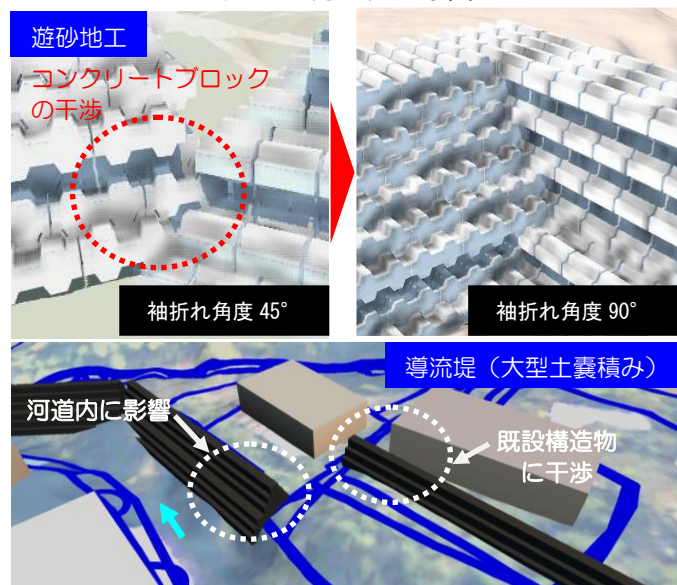
図-3 構造物の干渉チェック
