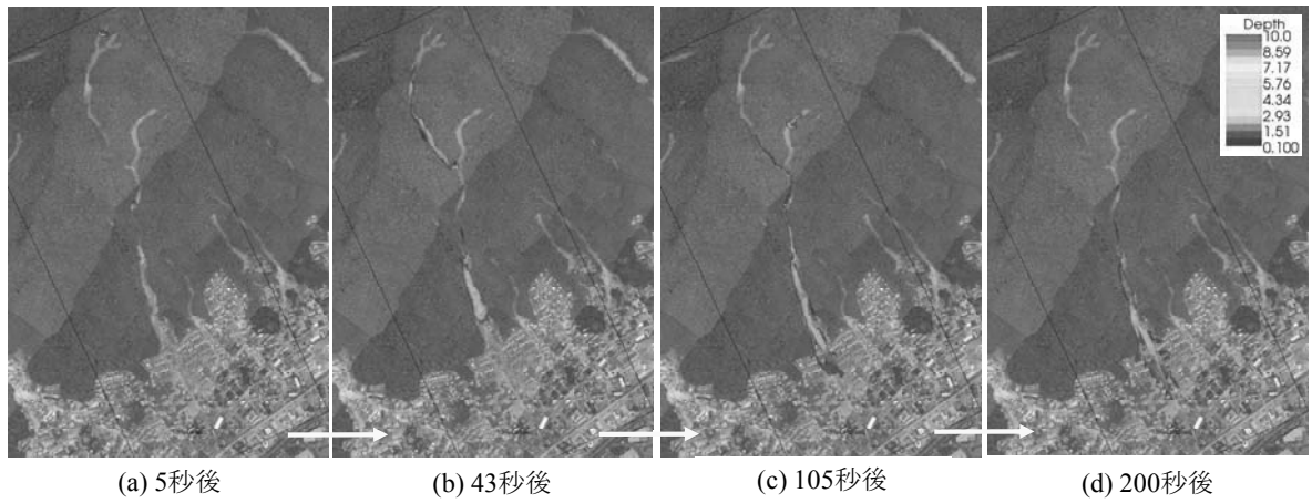
図2 流域全体の土石流の深さの時空間的な変化
