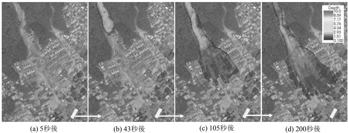
図4 家屋を考慮していない場合の住宅地の土石流の深さの時空間的な変化
