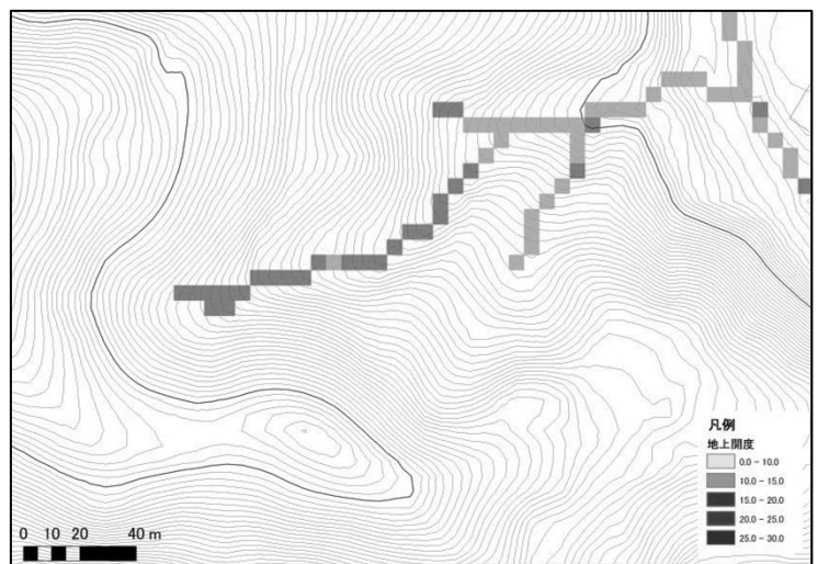
図 3 0 次谷渓流の谷形状と地上開度の関係（一例）
