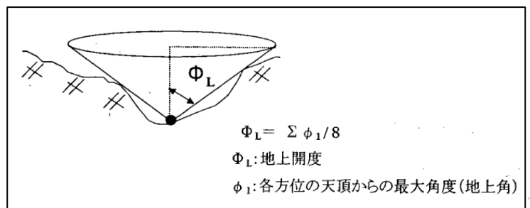
図 4 地上開度イメージ図 5)
