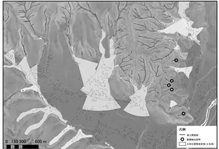
図 2 土石流に該当する新規箇所の抽出結果（一部抜粋）
