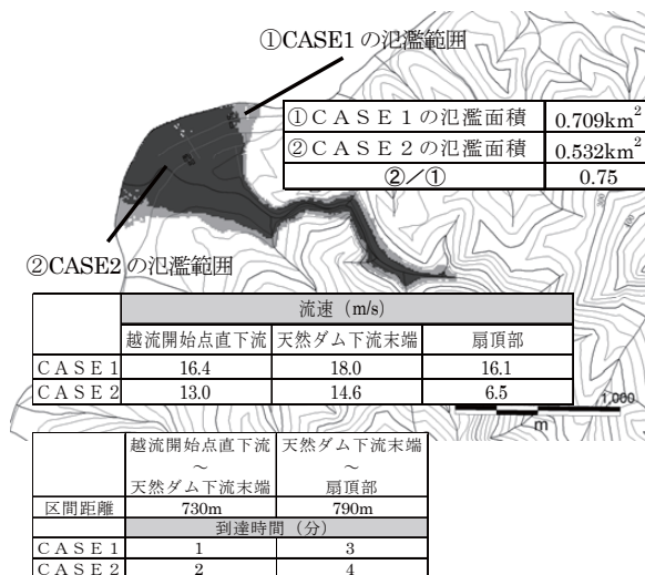
図-6 掘削前後の天然ダム決壊時の氾濫範囲の比較
