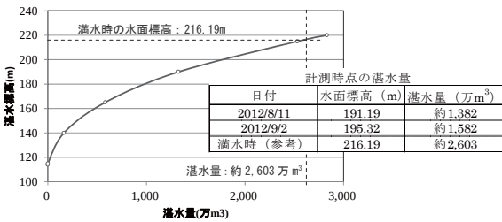
図-2 H-V 曲線
