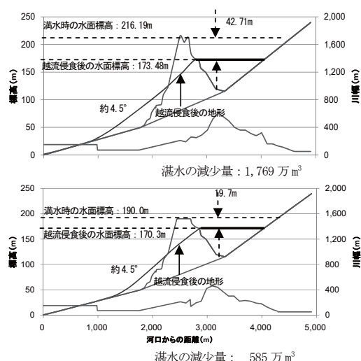
図-4 越流侵食による形状の変化 (上：CASE1、下：CASE2)
