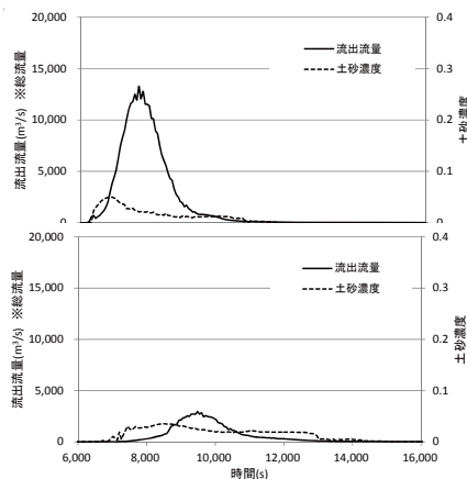
図-5 天然ダム下流のハイドログラフ (上：CASE1、下：CASE2)
