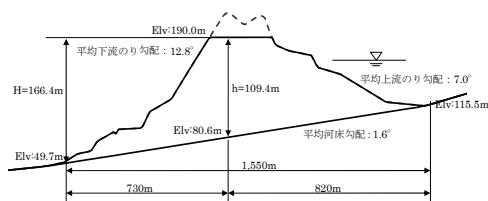
図-3 天端を開削した天然ダムの縦断形状
