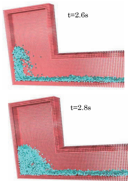
図-3 解析による流動状況
