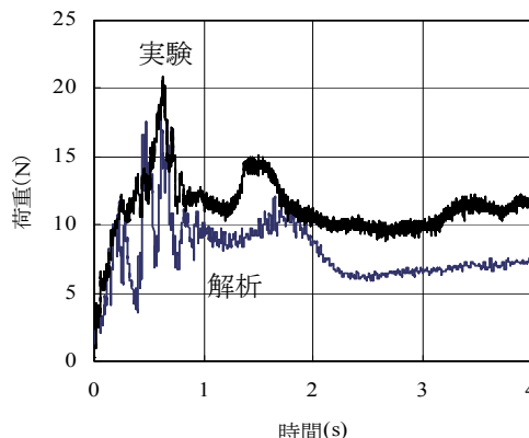
図-4 荷重～時間関係の比較
