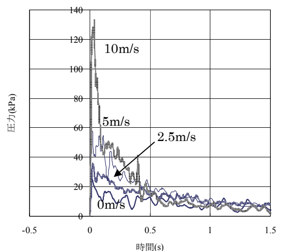
図-7 圧力～時間関係の比較
