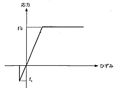
図-2 INSEM材の材料モデル
