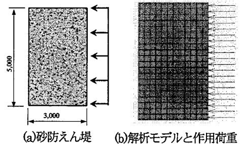
図-1 解析モデルと作用荷重
