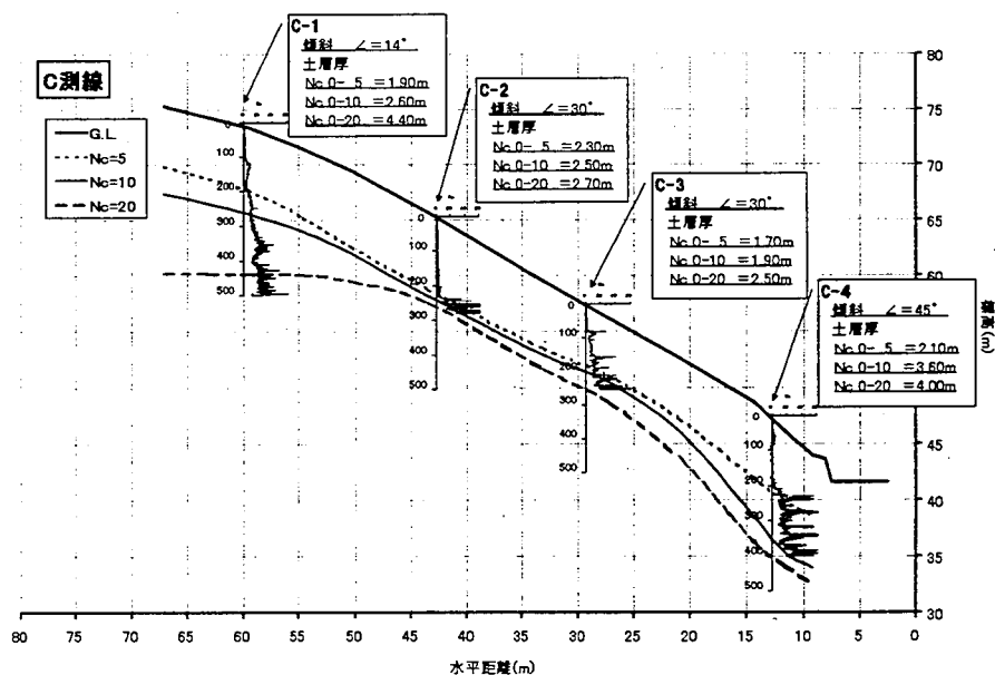
図3 推定土層厚断面図(C測線)
