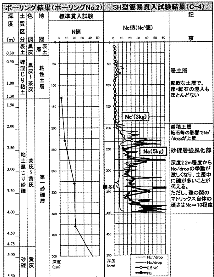
図2 ボーリング結果との対比
