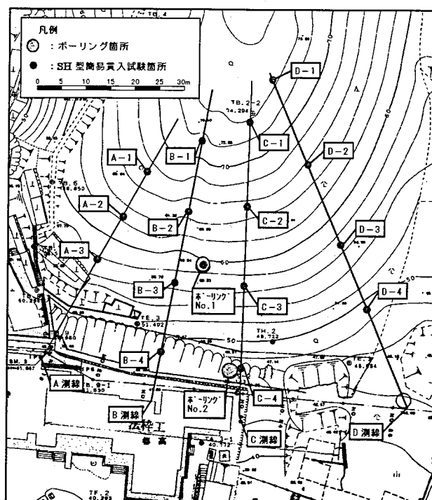
図1 調査地及び貫入試験位置図
