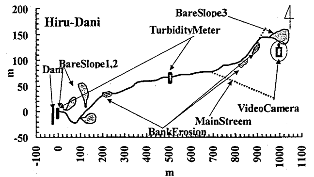
図1 観測流域平面図
