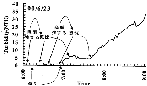
図4 裸地3付近での土砂供給イベントとダム地点の濁度変化
