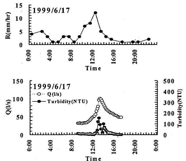
図3 一洪水中の降雨量、流量およびダム付近の濁度変化
