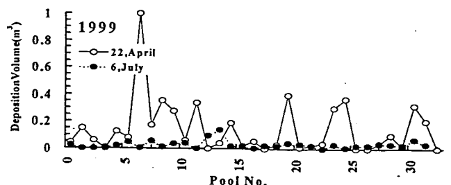
図6 プール内の堆積土砂量の変化
