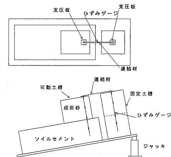
図2-1 試験装置概要
