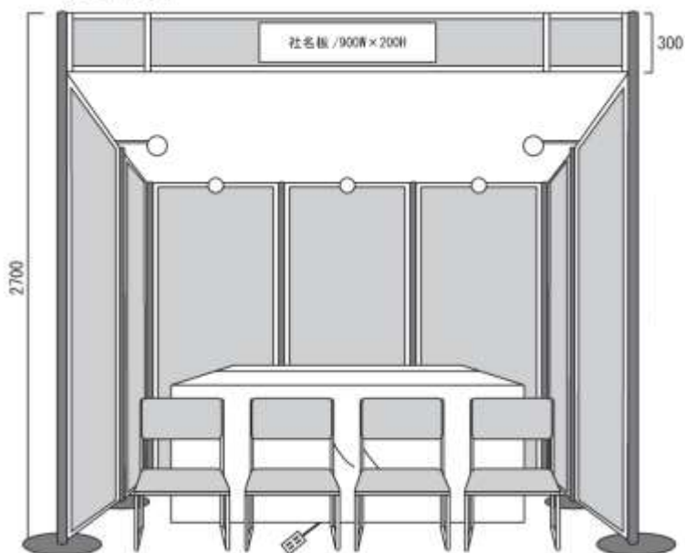
【立体図】
