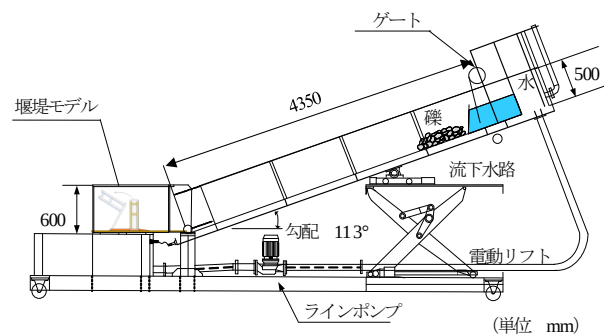
図-2 可変勾配型直線水路
