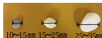
写真-2 供試体
