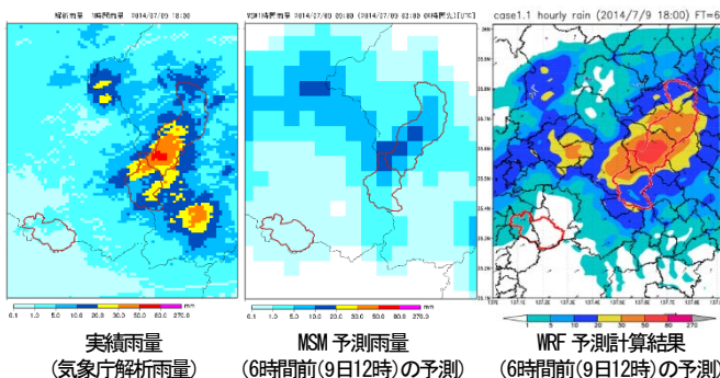
図-6 南木曽土石流災害時(7月9日18時)の実績雨量、予測雨量
