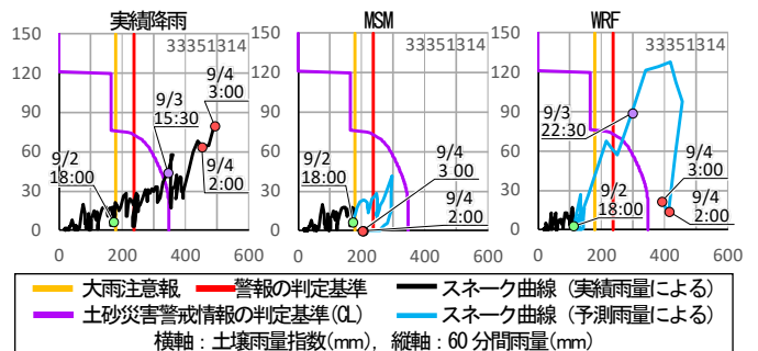
図-9 那智川土石流の実績降雨およびMSM, WRF (ともに32時間前(2日18時)での予測)によるスネーク曲線
