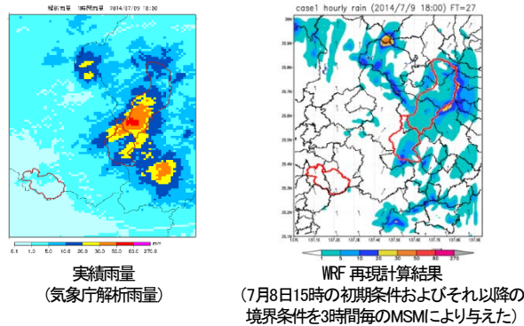
図-4 南木曽土石流の解析降雨とWRFによる再現計算結果 (平成26年(2014年)7月9日18時の時間雨量)
