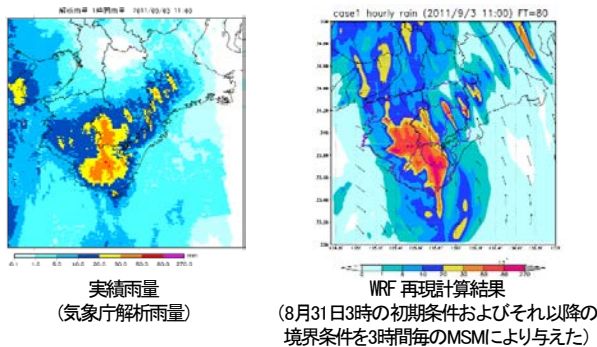
図-5 那智川土石流の解析降雨とWRFによる再現計算結果 (平成23年(2011年)9月3日11時の時間雨量)
