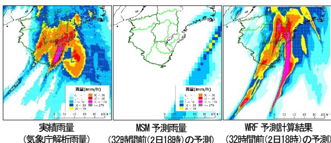
図-7 那智川土石流災害時(9月4日2時)の実績雨量、予測雨量
