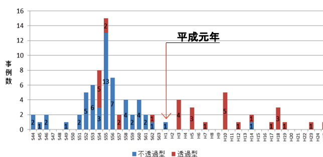
図－2 鋼材を用いた砂防施設の変状施設数
