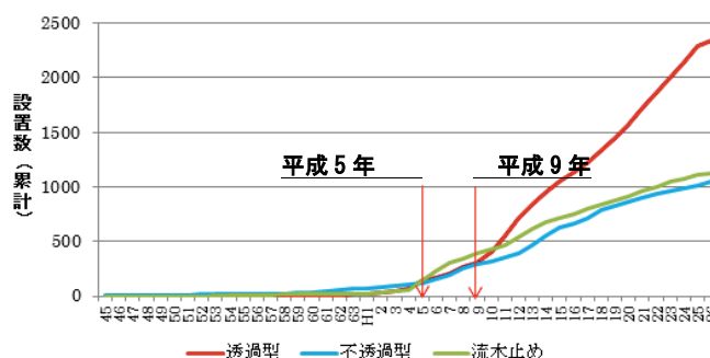
図－1 鋼材を用いた砂防施設の設置数
