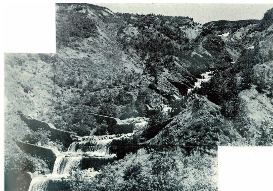
写真 1 甚之助谷階段式堰堤群 (S37 撮影)
