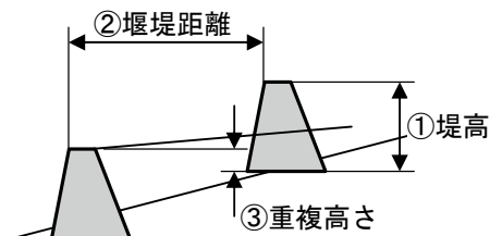
図 1 階段式堰堤群の特徴
