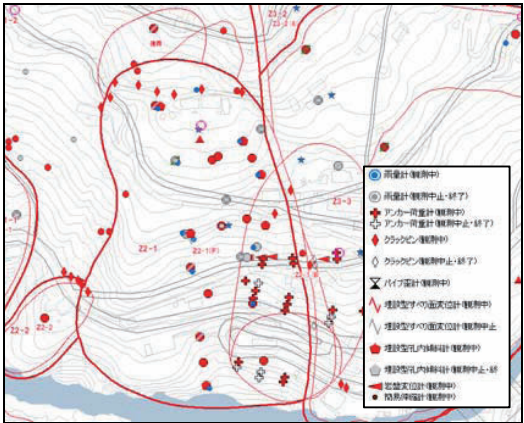
図-3 地滑り観測機器位置情報
