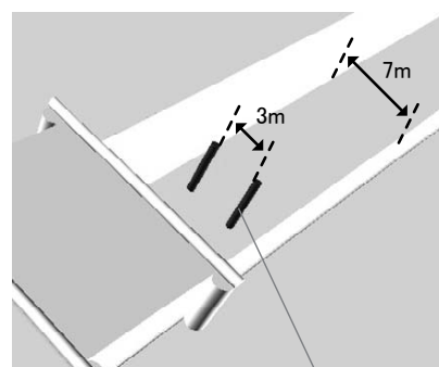
流木捕捉工
