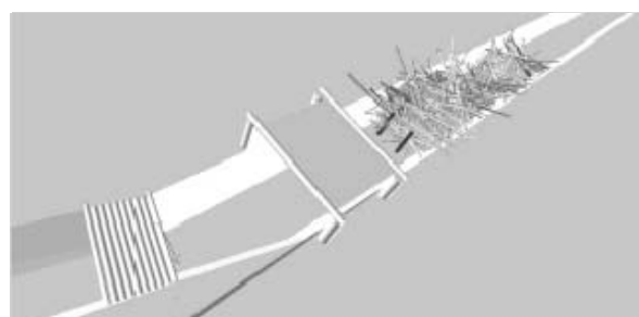
図-6 流木捕捉工を設置した解析結果 (流量 110 \text{m}^3/\text{s} ，流下密度 2.8 本/s)
