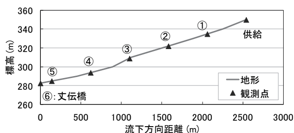
図-1 縦断断面図と流量解析の観測点
