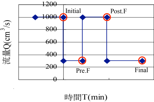
図-3 流量ハイドログラフ
