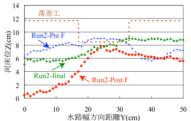
図-6 落差工上流部の横断形状 ( X=2.0(\text{cm}) )
