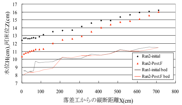
図-4 水路中央部の水位・河床位の縦断
