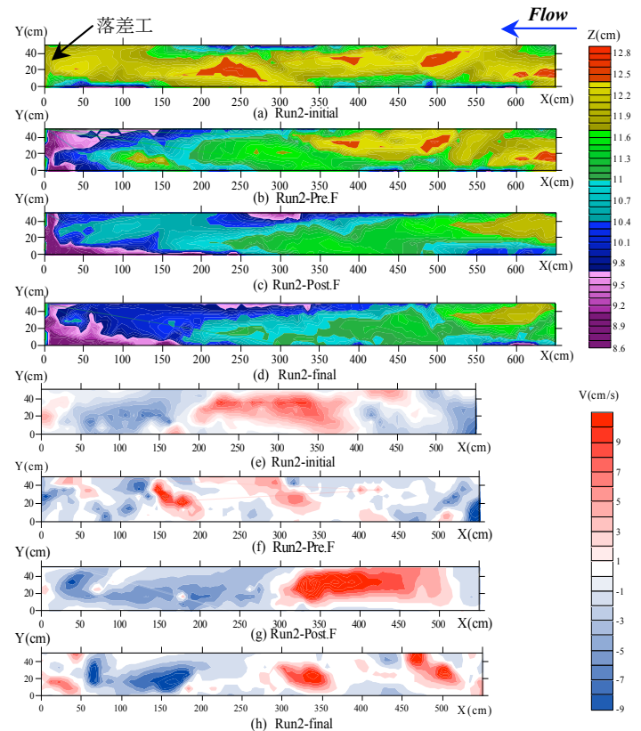
図-5 河床形状と横断方向流速 V の対応関
