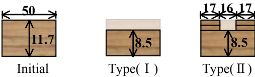
図-2 落差工模型の形状(単位:cm)
