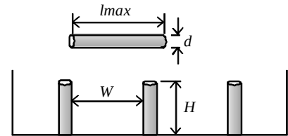
図-1 捕捉工の間隔と最大流木長
