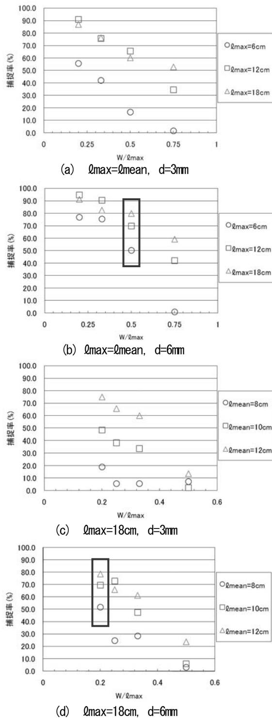
図-2 流木捕捉率～ W/l_{max} 関係
