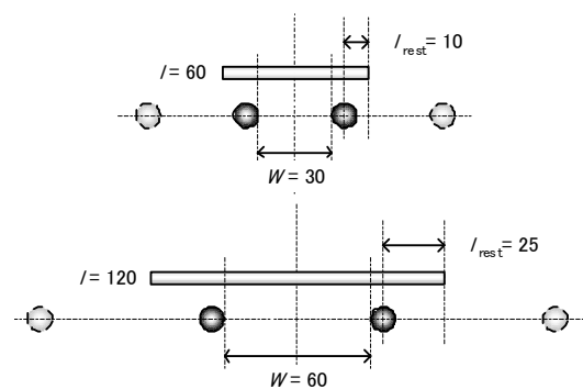
図-3 流木長ごとの余長 l_{rest}
