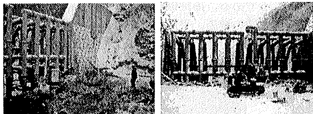
写真3 索道による除石の事例
