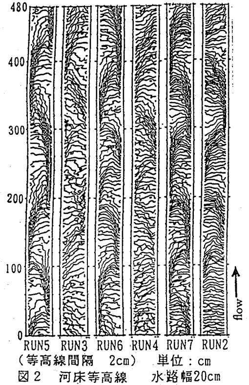
図2 河床等高線 水路幅20cm
