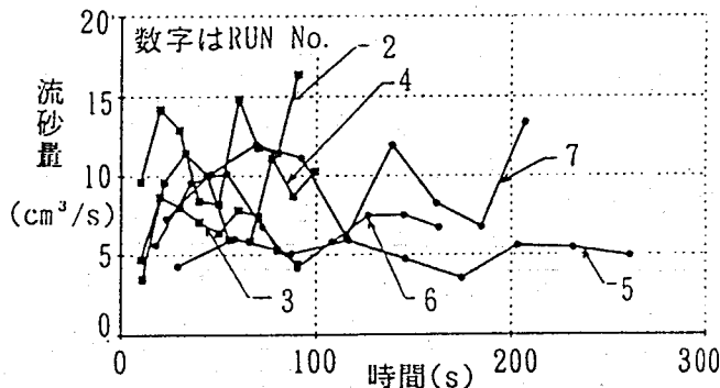
図4 流砂量の時間的変動
