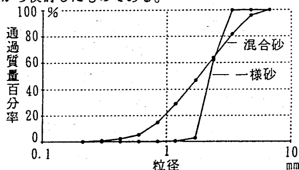
図1 河床材料の粒度分布
