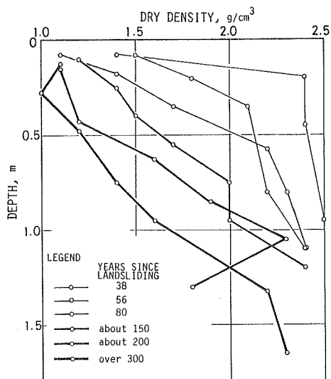
図5 乾燥密度の経年変化
