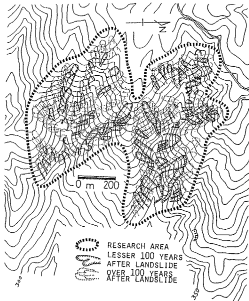
図2 山くずれの分布
