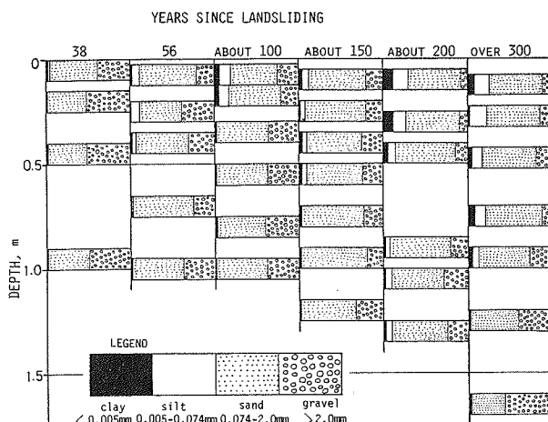
図6 粒度の経年変化
